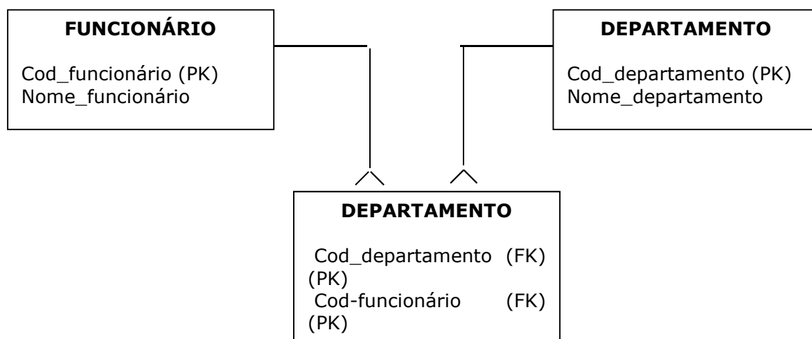
FIGURA 1 – MODELO RELACIONAL NORMALIZADO
